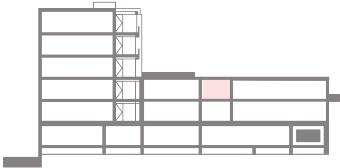
TYPE DV1 DOORSNEDE A-AT
