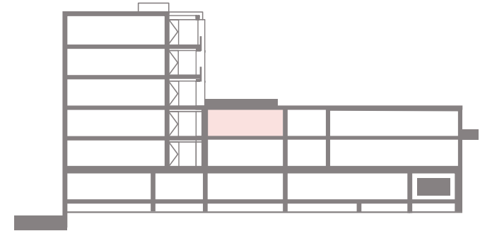
YPE E V1 DOORSNEDE A-A
