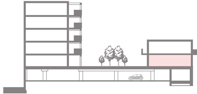
TYPE C DOORSNEDE B-B
