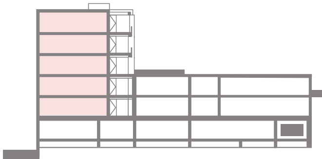
TYPE F DOORSNEDE A-AT
