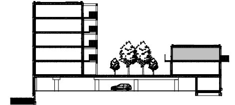
doorsnede B-B
