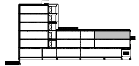
doorsnede A-A
