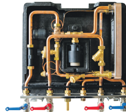
Aansluiting warmtenet.
